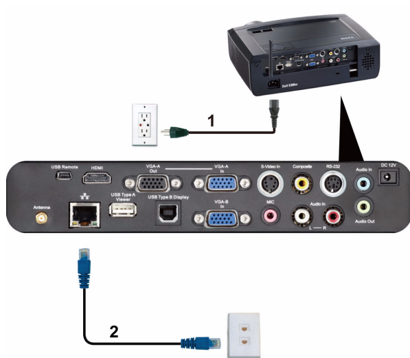
Локальная вычислительная сеть (ЛВС)
